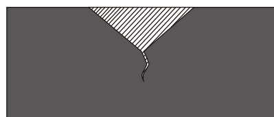
クラックのVカット補修
